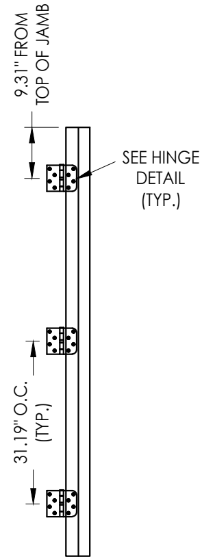
HINGE JAMB
